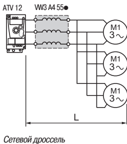
Сетевой дроссель
