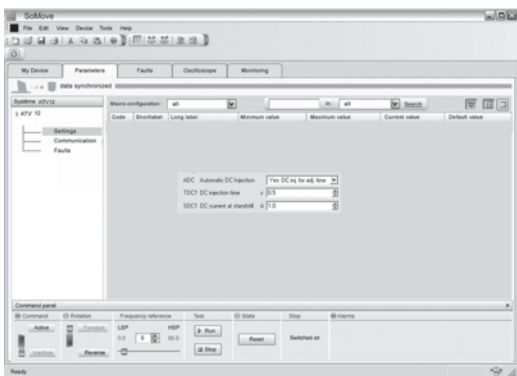
Настройка функции торможения постоянным током с помощью программного обеспечения SoMove
