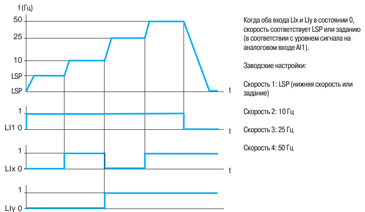
Пример работы с 4 заданными скоростями
