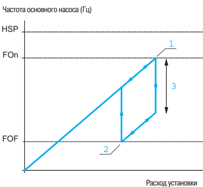
Работа основного и вспомогательного насосов: гистерезис
