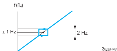
Пропуск частотного окна относительно резонансной точки
